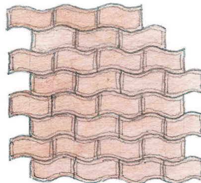
FIG. 4 - PIASTRELLE AUTOBLOCCANTI IN CLS COLORATE
